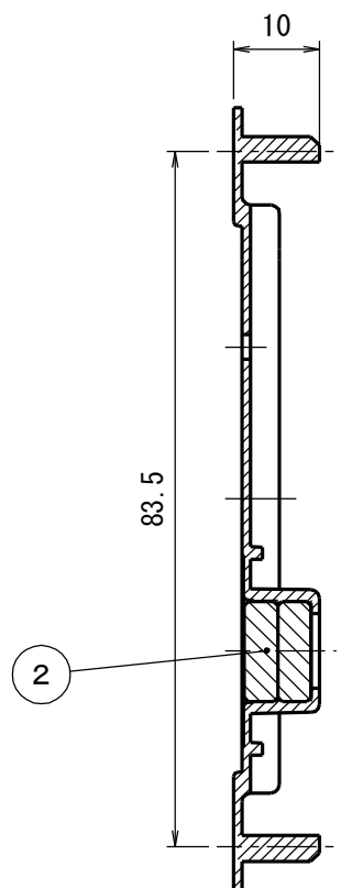
A-A断面図
